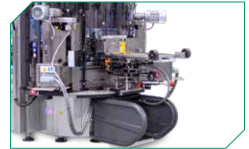
Station d'étiquetage colle à chaud pour applications enveloppantes en papier.
